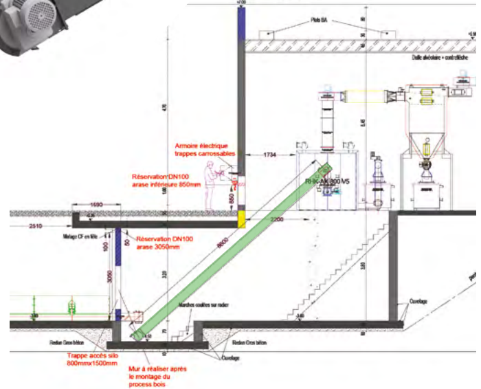
COUPE 2-2
